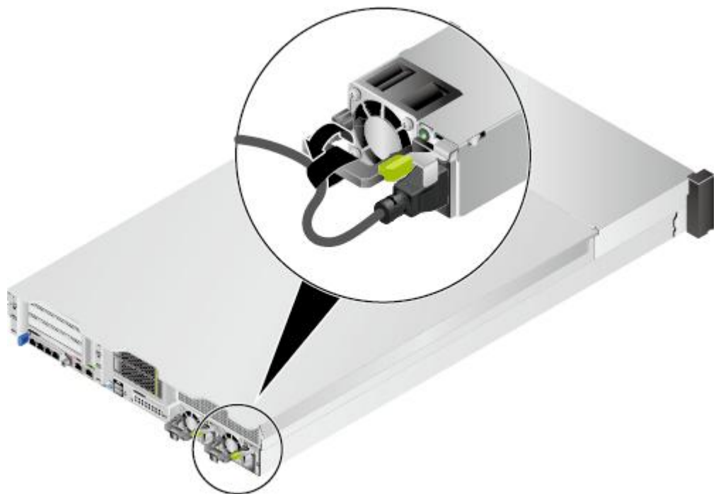
图 6-16 固定电源线缆
