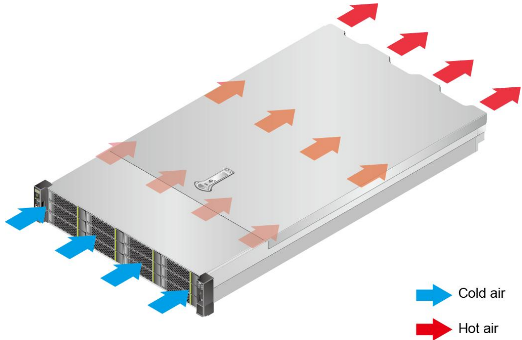
图 6-4 散热气流走向示意图
