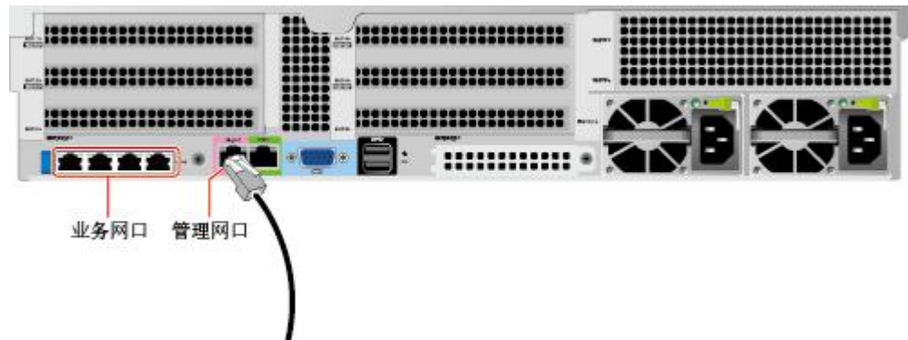
图 6-12 连接网线
