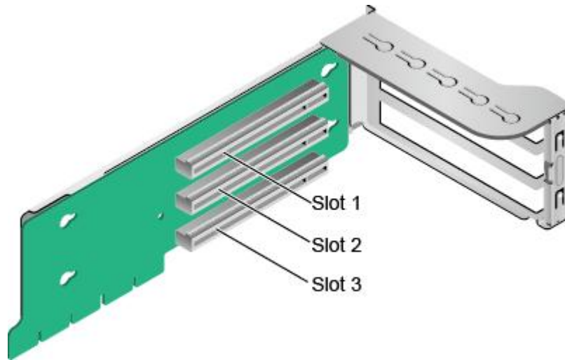
图 3-9 Riser 卡 1 (3x8)
