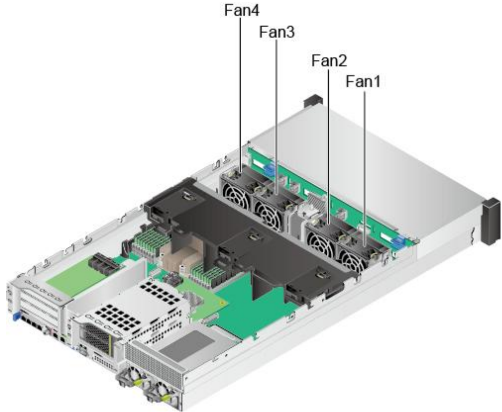
图 3-13 风扇位置图
