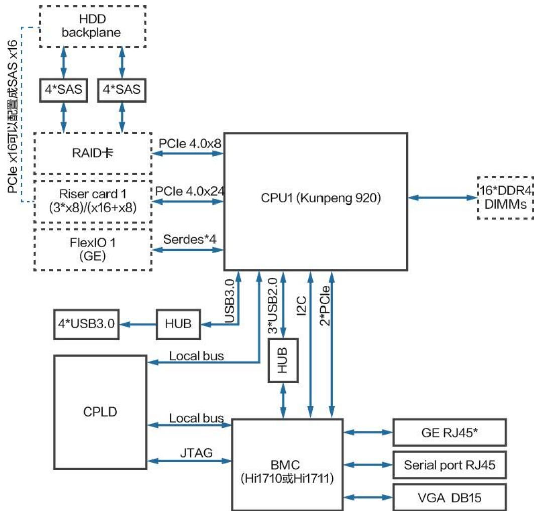
图 2-3 逻辑结构 (配置鲲鹏 920 7260 或 5250 处理器)
