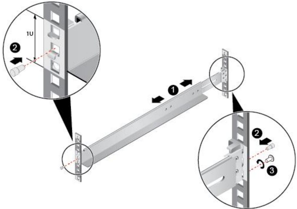
图 6-9 安装可伸缩滑道
