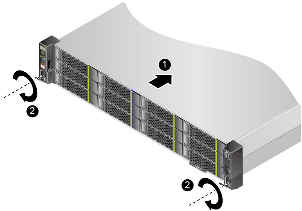
图 6-8 安装服务器
