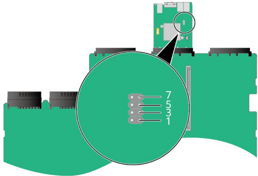
图 8-14 跳线位置
