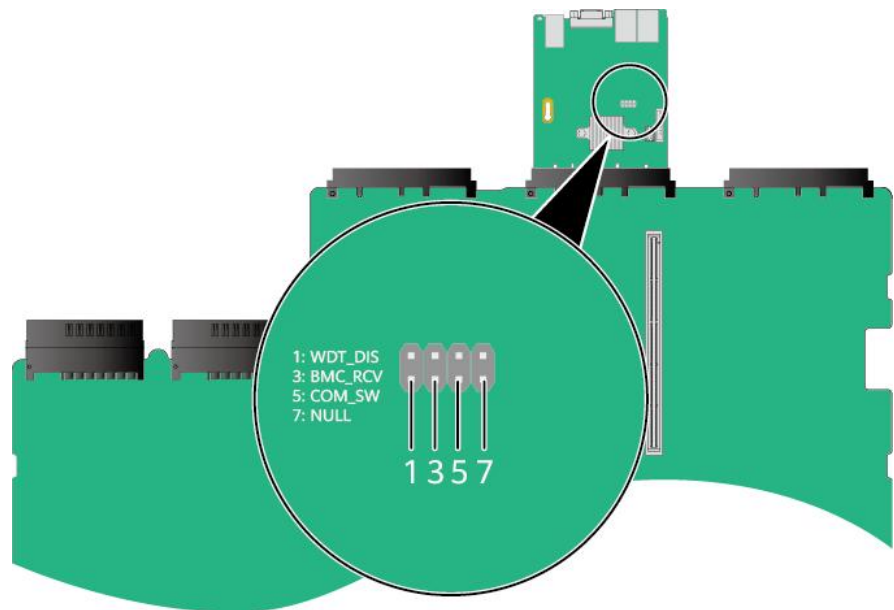
图 8-13 跳线位置
