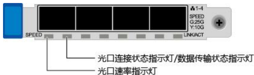
图 3-6 TM280（4x25GE 光口）
