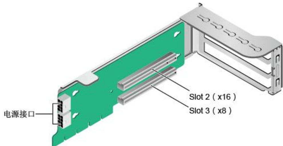
图 3-10 Riser 卡 2 (1x8+1x16)
