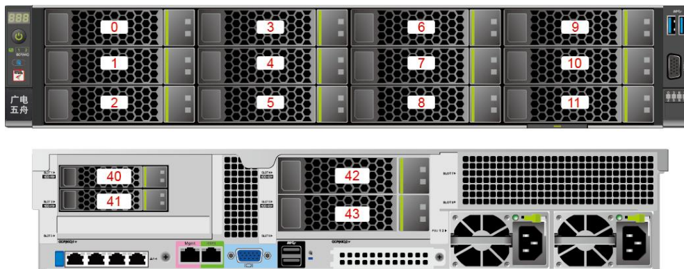
图 3-7 12x3.5 英寸硬盘 EXP 配置硬盘编号
