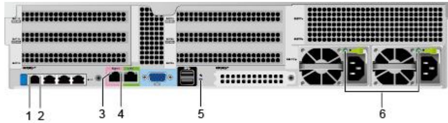
图 3-4 后面板指示灯
