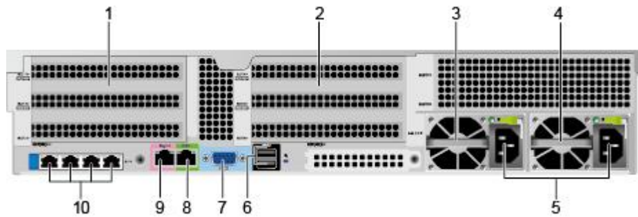
图 3-3 后面板组件
