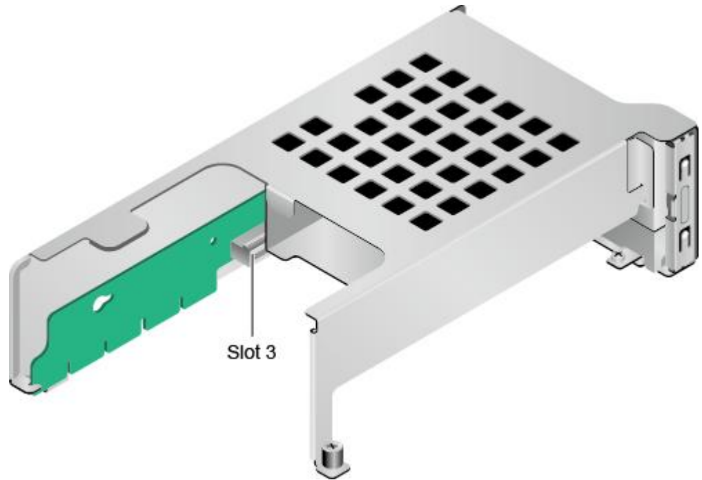
图 3-11 Riser 卡 3 (1x16)
