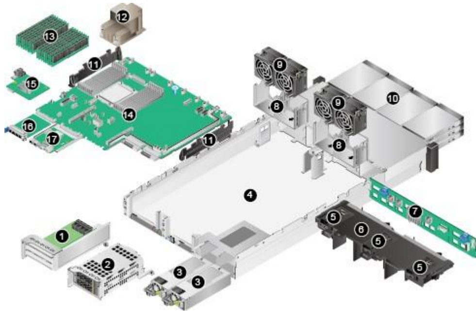
图 2-2 部件（配置鲲鹏 920 7260 或 5250 处理器）
