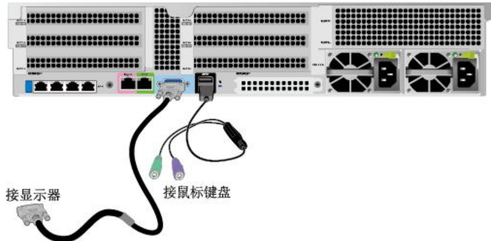
图 6-11 连接 USB 转 PS2 线缆和 VGA 接口
